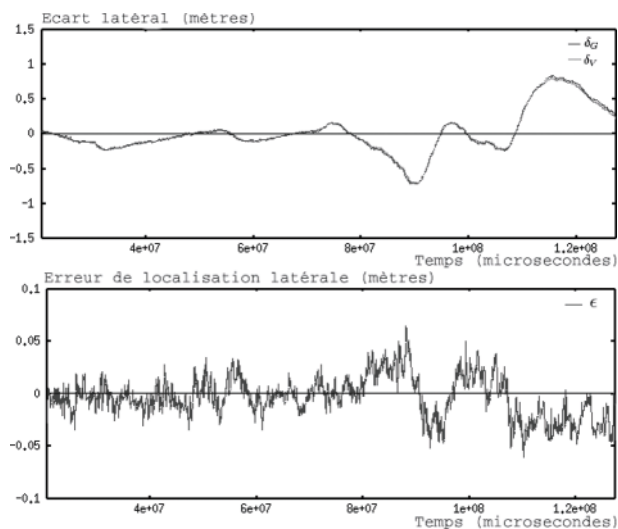
Figure 9. Erreur latérale (en haut) mesurée avec le GPS \delta_G (bleu) ou par vision \delta_V (rouge) et erreur de localisation latérale \epsilon (bas).
