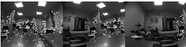
Figure 15. De gauche à droite images prises à 0^\circ , 44^\circ et 90^\circ , avec les points d'intérêt correctement appariés en surimpression.
